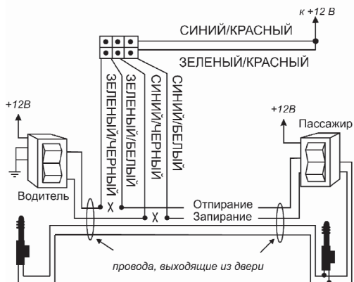
Схема 4 Однопроводный тип цепи дверных замков с отрицательной полярностью (некоторые автомобили марки Ниссан, Mazda и др.)
